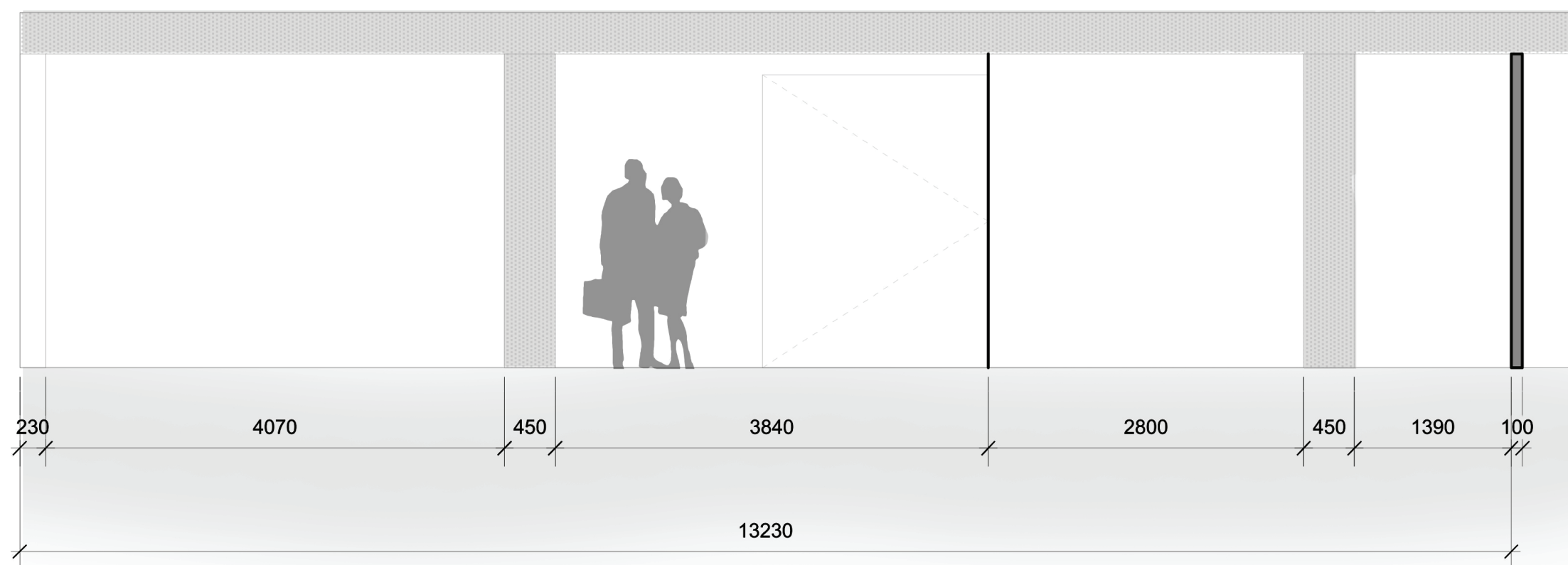
Space I - Section 'BB'
